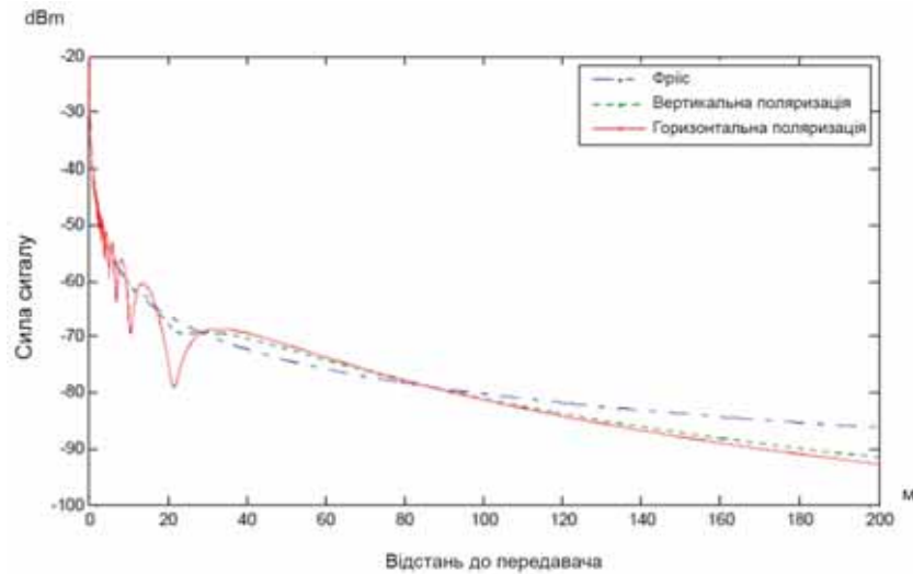
Рис. 2. Втрати при передачі відповідно до поляризації сигналу
