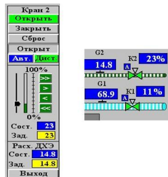
Рис. 7. Фрагменти мнемосхем керування виконавчими пристроями
