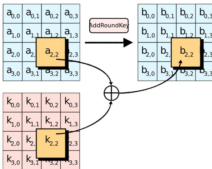
Рис. 4 - Процедура AddRoundKey
