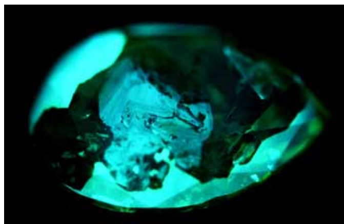
Рисунок 4. Діамант жовто-зеленого кольору під час опромінення УФ-хвилями в приладі "DiamondView™", \lambda_{\text{випр.}} < 225 \text{ нм}
