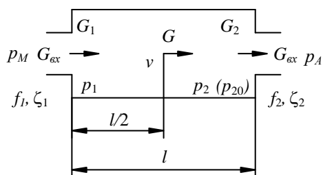
Рис. 4. Расчетная схема пневматической линии
