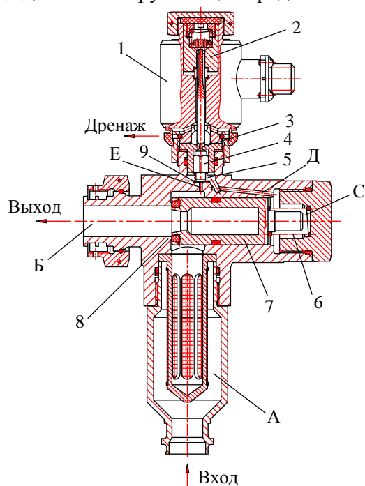
Рис. 1. Высокорасходный ЭПК: А, Б, С – входная, выходная и управляющая полости соответственно; Д, Е – каналы; 1 – электромагнит; 2 – якорь; 3 – дренажное седло; 4 – управляющий клапан; 5, 6 – пружины; 7 – основной клапан; 8 – седло основного клапана; 9 – впускное седло
