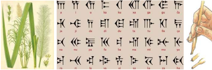
Рис. 2. Клинопис
