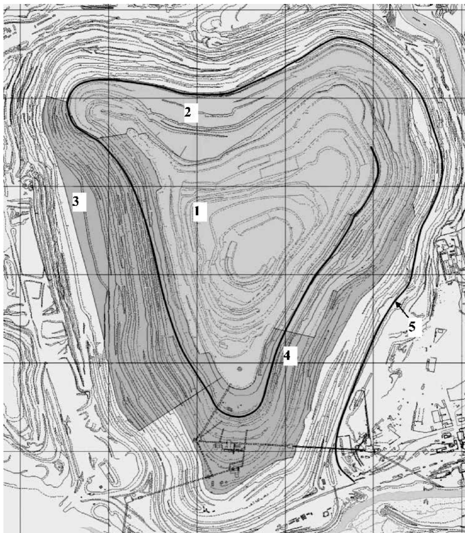
Рис. 1. Проект реконструкции транспортной схемы карьера ПАО «ЮГОК»:
