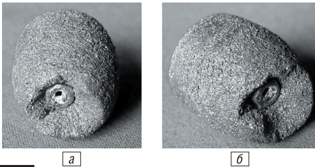
Рис. 14. Вид образцов проницаемого пористого железа, полученного путем АСД из прессованных (не спеченных) порошковых цилиндров исходным диаметром 12 мм; трансформация пористости от 15 до 65 %; увеличение прочности в 25 раз (в центре отверстие для заделки термопары)
