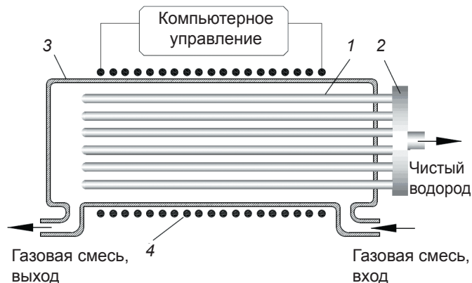
Рис. 16. Схема ячейки для промышленного получения чистого водорода из газовых смесей с использованием Н-слоев: 1 – железные (стальные) трубчатые мембраны; 2 – коллектор водорода; 3 – герметичный цилиндр из аустенитной стали; 4 – нагреватель
