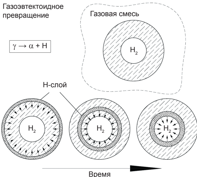
Рис. 15. Схема работы Н-слоев в трубчатой водородной мембране
