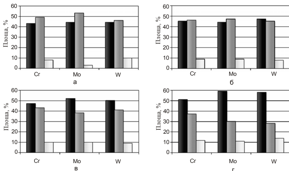
Рис. 6. Співвідношення площ у структурі сталі P6M5 з мінімальним, середнім та максимальним вмістом легуючого елемента після переплаву при різних температурах нагріву розплаву T_n . а – T_n = 1460 °C, б – T_n = 1500 °C, в – T_n = 1540 °C, г – T_n = 1620 °C.
