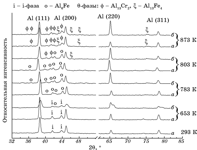
Рис. 2. Спектры рентгеновской дифракции порошка (кривые a ) и экструдированных образцов сплава Al 94 Fe 3 Cr 3 (кривые b ) до и после отжига при различных температурах в течение 30 мин.
