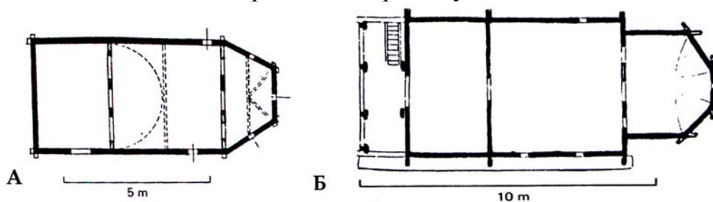
Рис. 1. Характерні плани румунських церков. А – церква з Куасені (Лапус), церква з Бростені (Горж), за Д. Букстоном
