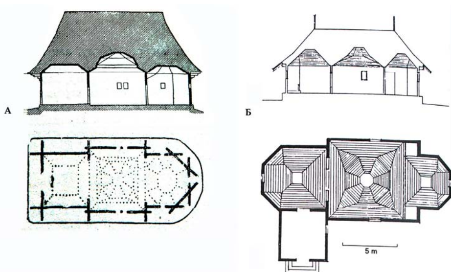
Рис. 4. Буковинські церкви з заломами. А – Церква св. Михайла, Чернівці (за Г. Логвіним); Б – Церква з села Дорогой, Румунія (за Д. Букстоном)
