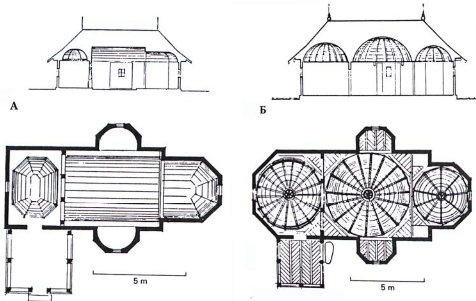
Рис. 5. Буковинські церкви без заломів (Румунія). А – Церква з Браїєшти; Б – Церква з Сервієшти (за Д. Букстоном)
