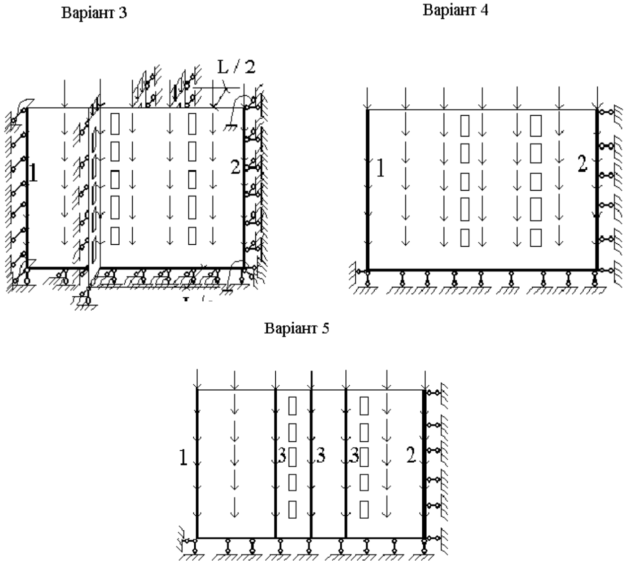
Рис. 2. - Схематичне зображення розрахункових схем третього, четвертого та п'ятого варіантів розрахунку: 1, 2, 3 - стрижневі КЕ, що моделюють поперечні стіни будівлі.
