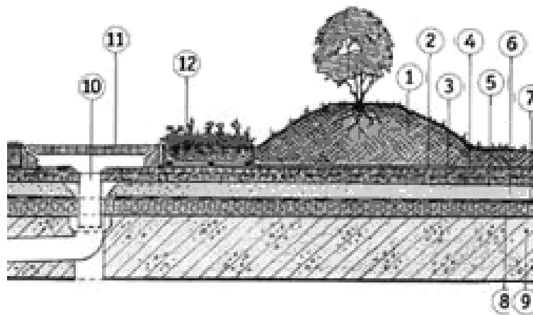
Рис. 3. Конструкція інтенсивного саду на даху: 1 – рослинний шар; 2 – фільтрувальний шар; 3 – дренажний шар; 4 – рівень води; 5 – протикореневий шар; 6 – вирівнюючий шар; 7 – гідроізоляція; 8 – теплоізоляція; 9 – залізобетонні плити; 10 – водостічна воронка; 11 – доріжка з решіткою для регулювання стоку води; 12 – контейнер для квітів вдовж доріжки.
