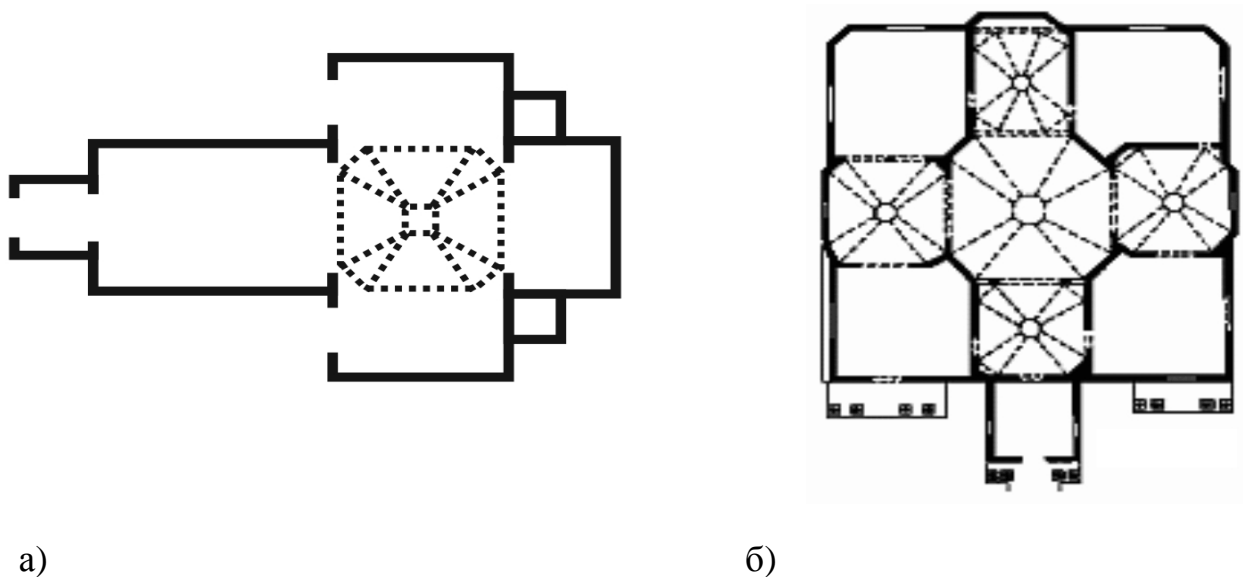
Рис. 4. Планування приміщень храмів у вигляді хреста а) схема плану церкви Покрови в с. Писарівка; б) схема плану церкви Св. Михайла в с. Дашів
