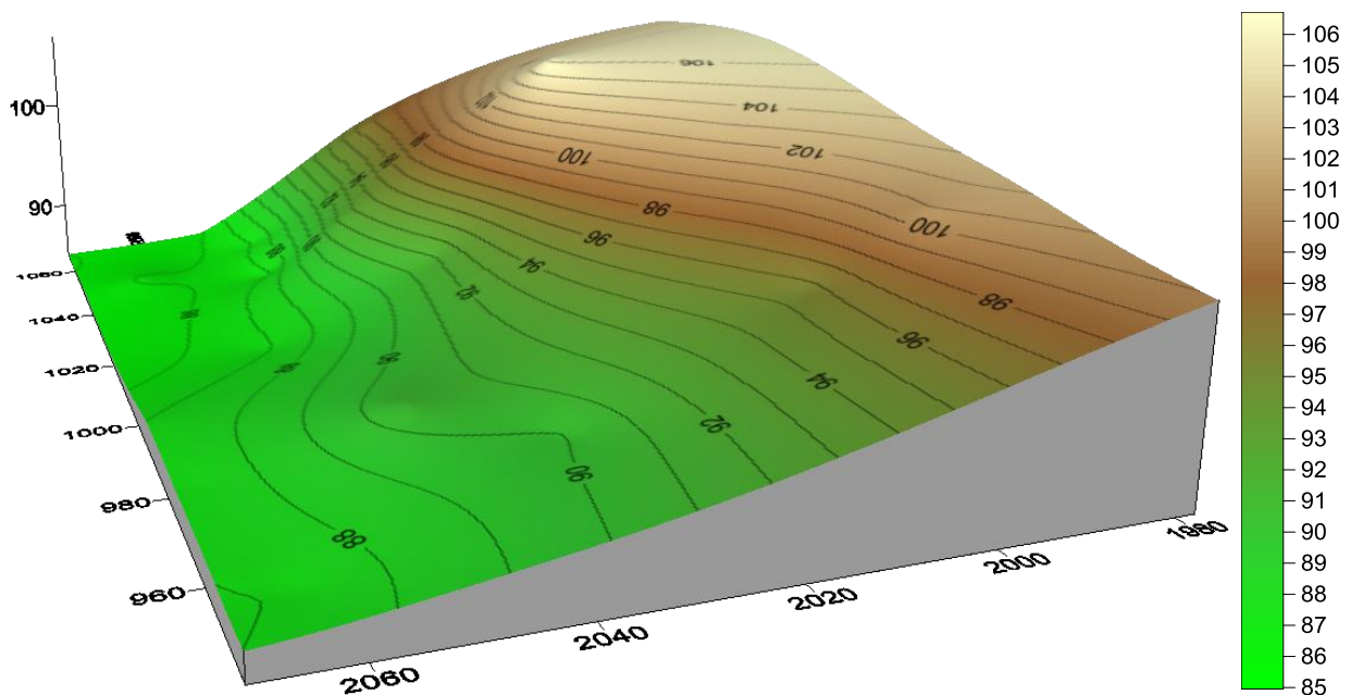
Рис. 4 Тривимірна модель поверхні зсуву
