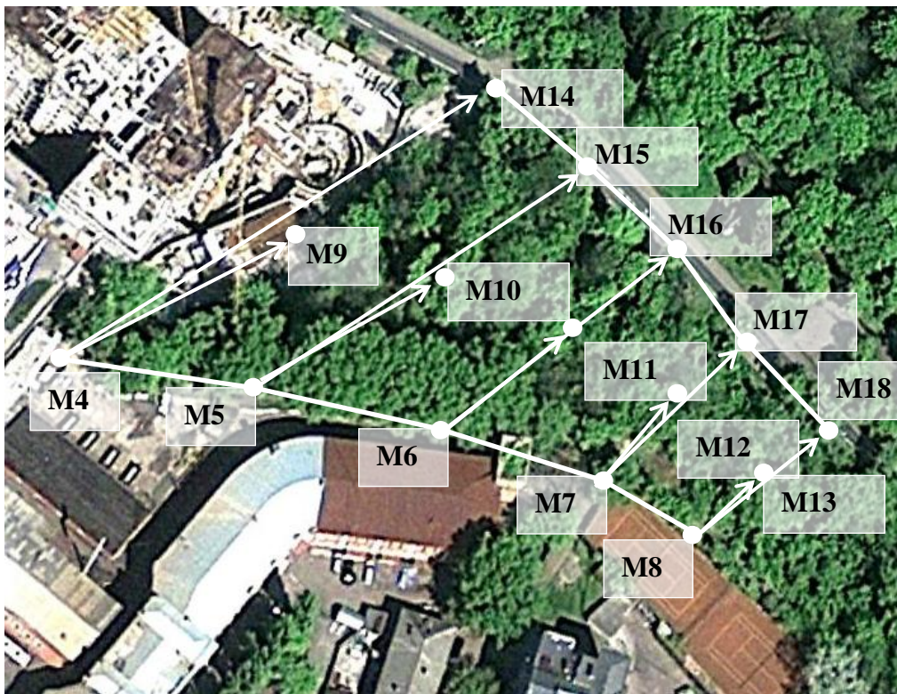
Рис. 2. Проектна мережа станцій спостережень
