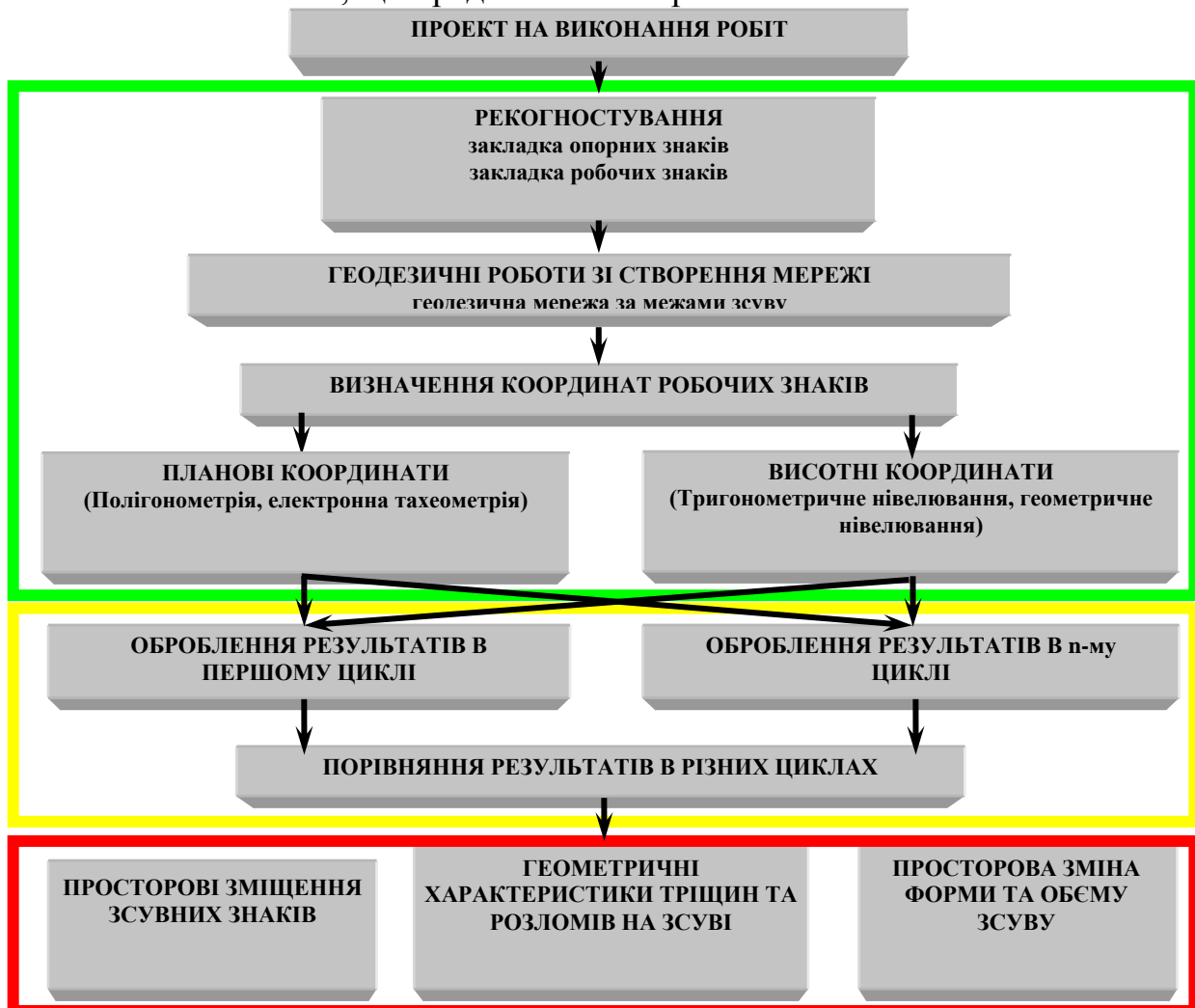
Рис. 1. Технологічна схема спостереження за зсувами
