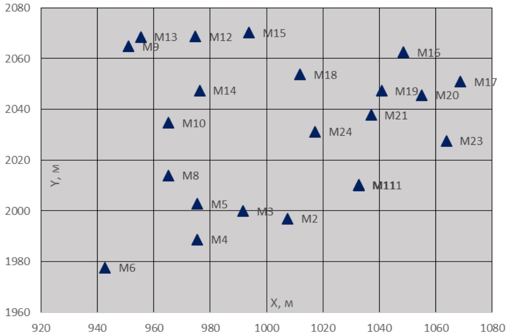
Рис. 3. Робоча мережа станцій спостережень
