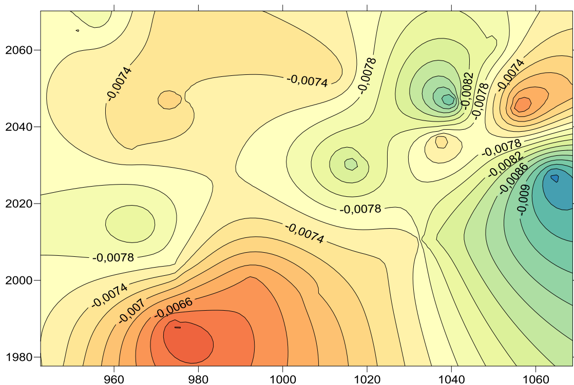
Рис. 5 Рельєф композитної поверхні деформацій зсуву
