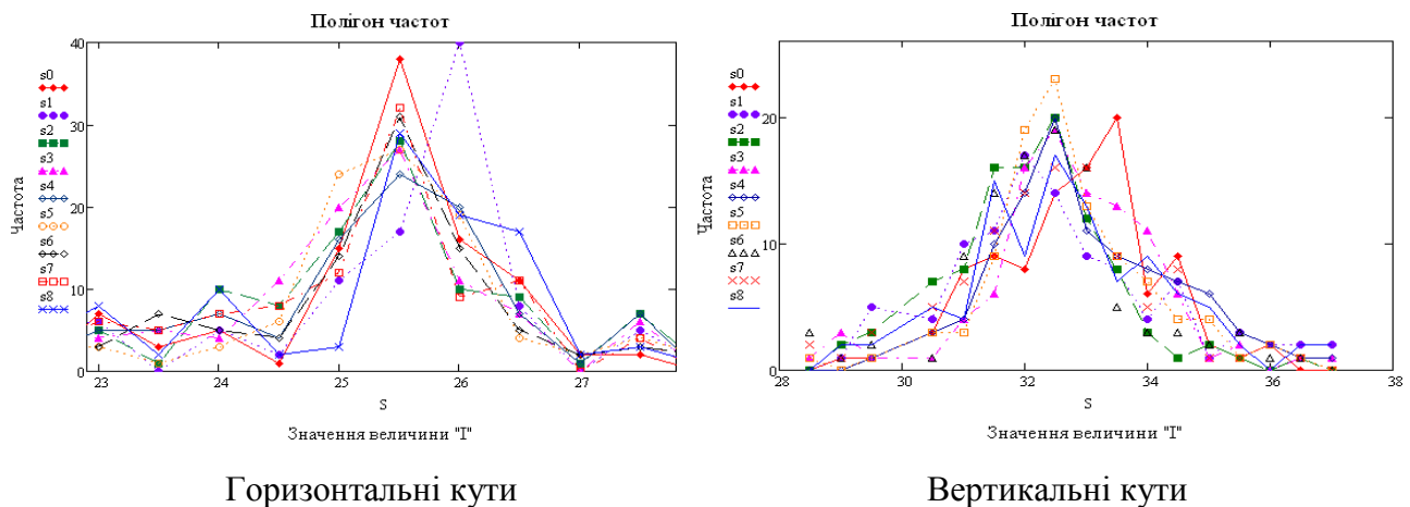
Рис. 1.2 Полігони частот варіаційних рядів
