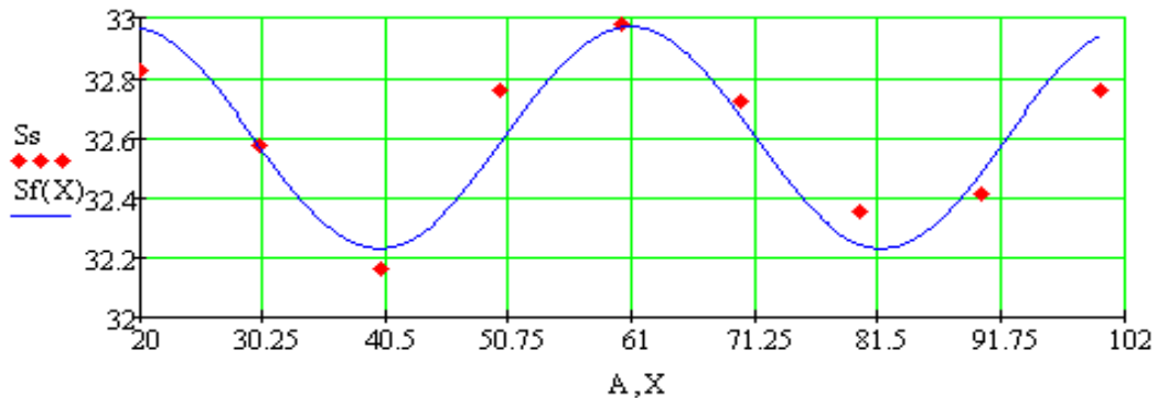
Рис.1.8 Синусоїдальна залежність між частотою і амплітудою вертикальних кутів
