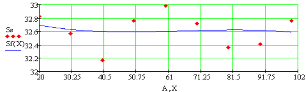
Рис.1.6 Математична залежність поліномом 3-ї степені вертикальних кутів
