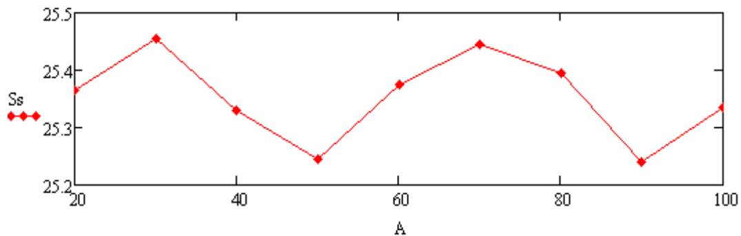
Рис. 1.3 Оцінка характеру математичної залежності для горизонтальних кутів
