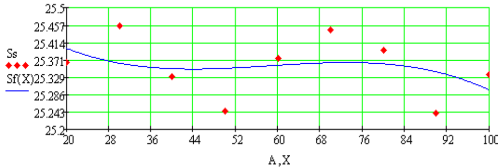
Рис.1.5 Математична залежність поліномом 3-ї степені горизонтальних кутів
