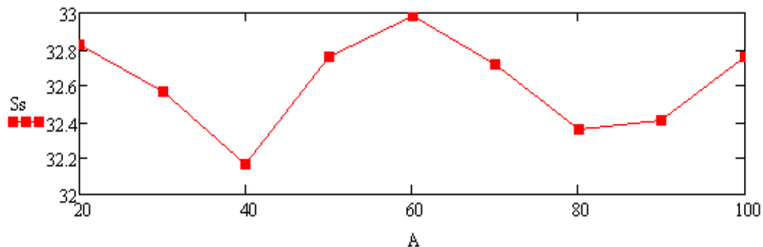
Рис. 1.4 Оцінка характеру математичної залежності для вертикальних кутів
