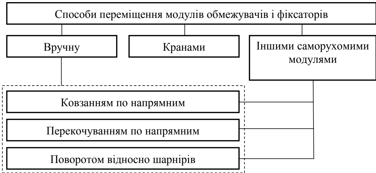
Рис.3. Класифікація способів переміщення модулів оснастки
