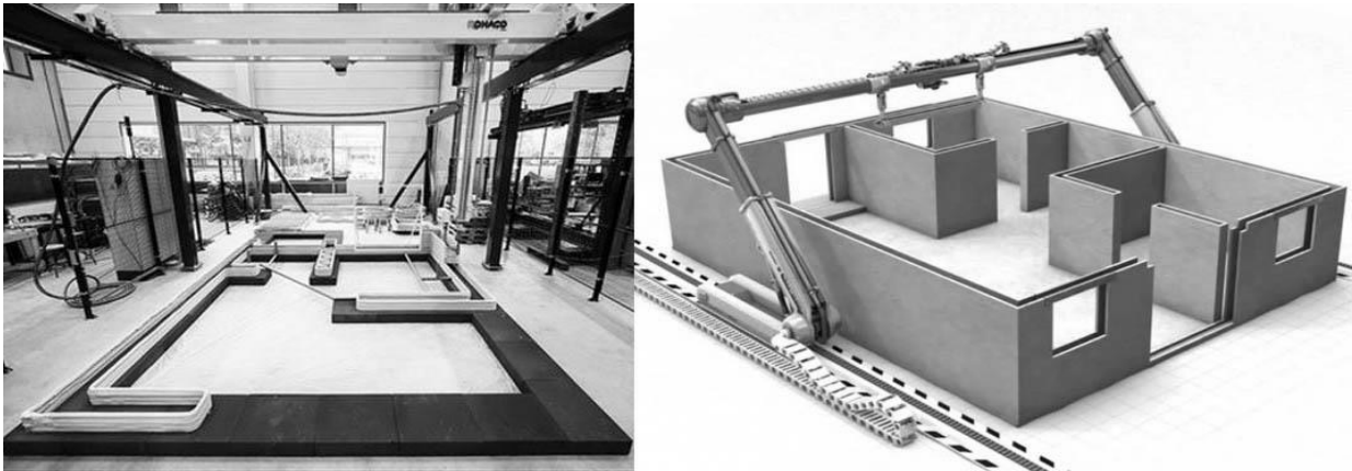
Мал. 2. Варіанти розповсюдженої конструкції будівельних 3D принтерів. Принтер «Contour Crafting» професора Берока Хошневіса з університету Південної Каліфорнії, США (справа).
