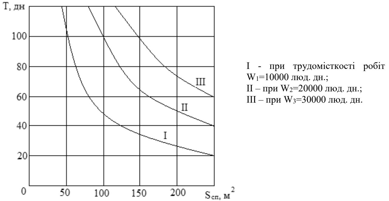
Рис.2. Залежність площі гардеробних S_{сп} від тривалості робіт T ( e=0,55 )
