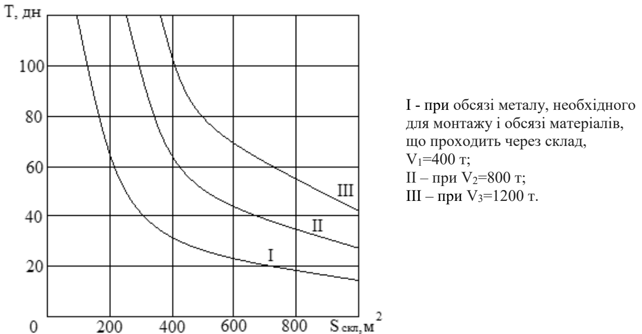
Рис.1. Залежність площі відкритих складів металоконструкцій S_{\text{скл}} , що транспортуються на відстань менш 50 км, від тривалості робіт T ( e=0,03 )
