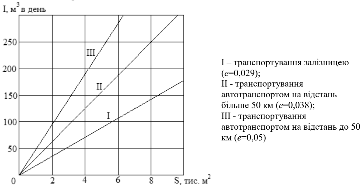
Рис. 3. Залежність площі відкритих складів збірних залізобетонних конструкцій від інтенсивності робіт
