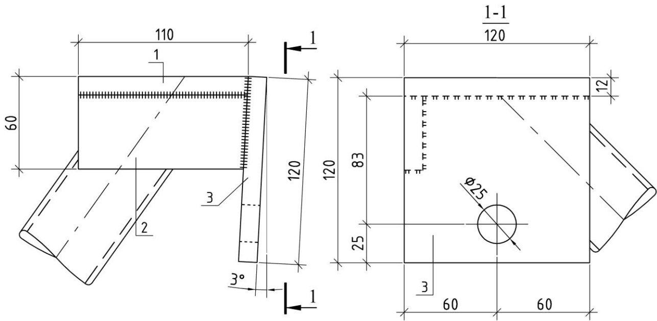
Рисунок 5 – Деталь вузла з'єднання сталезалізобетонних модулів
