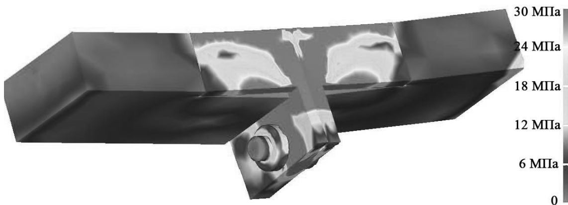
Рисунок 6 – Напружено-деформований стан вузла з'єднання
