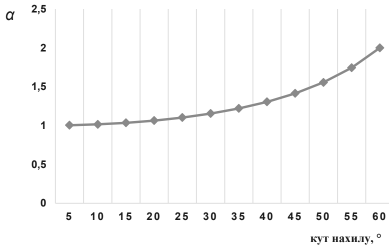
Рис. 1. Залежність площі покриття від кута нахилу покрівлі
