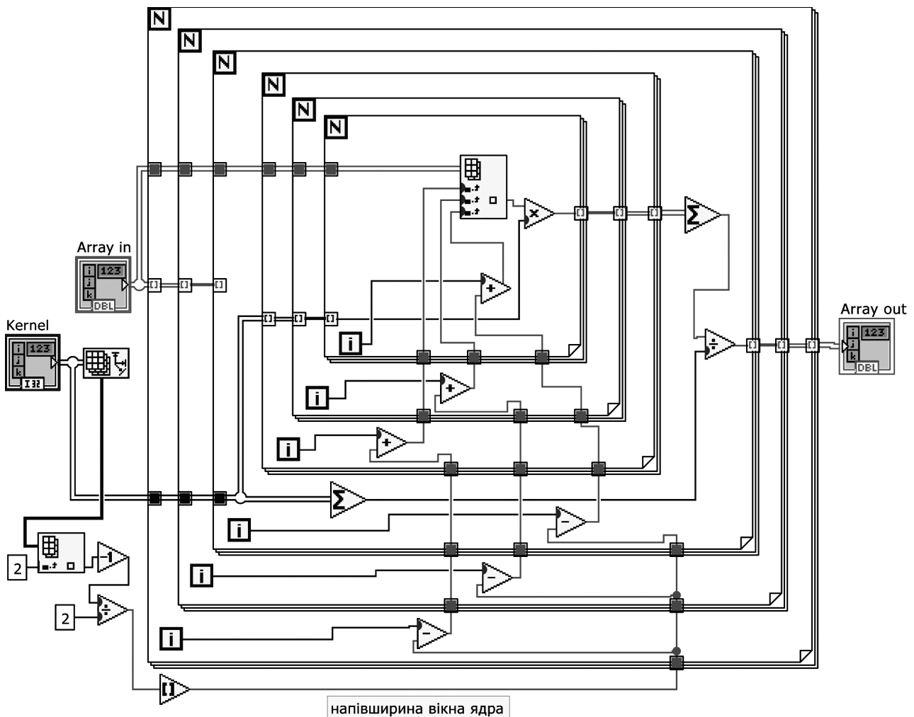
Рис. 1. 3-вимірний фільтр Гаусса для 3D-реконструктора
