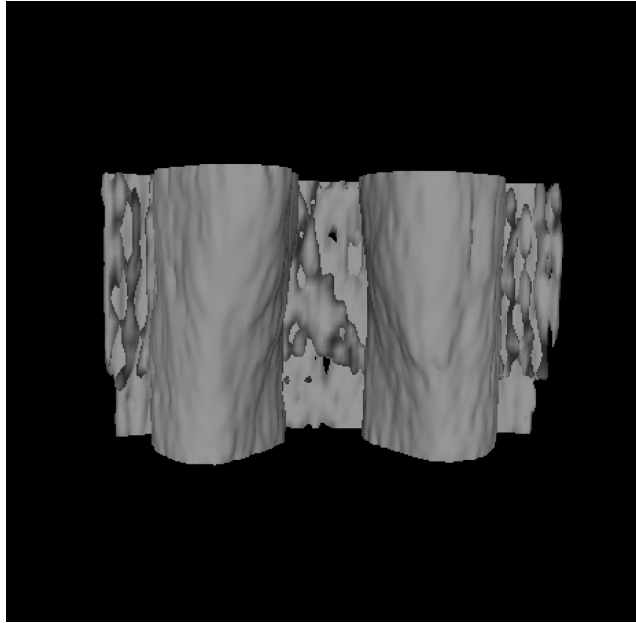
Рис. 2 – 3D-реконструкція фрагмента із застосуванням фільтра Гаусса
