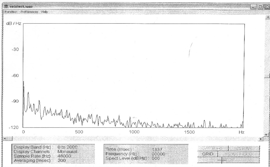
Рис.1. Спектр магнітного поля трамвайної лінії (відстань - 25 м)
