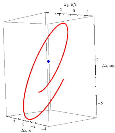
б) фазовий портрет руху системи для випадку 7
