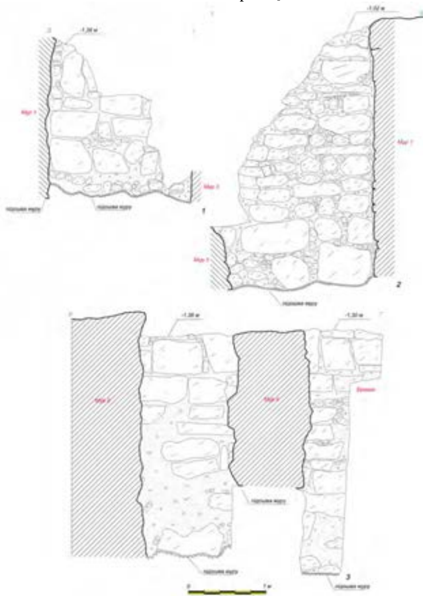
Рис. 7. Розгортки мурів: 1 – мур 4; 2 – мур 2; 3 – мур 1 Fig. 7. Scan of the walls: 1 – wall 4; 2 – wall 2; 3 – wall 1
