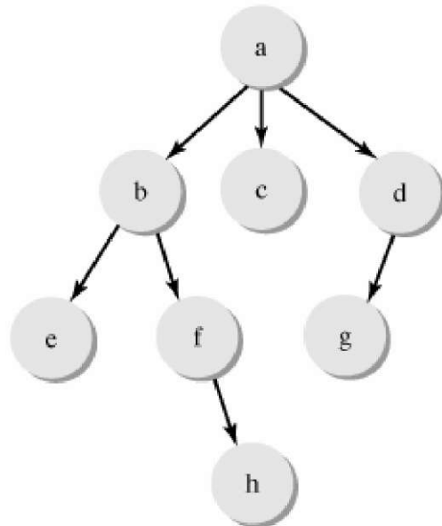
Рис. 4. Напрявлене дерево.
