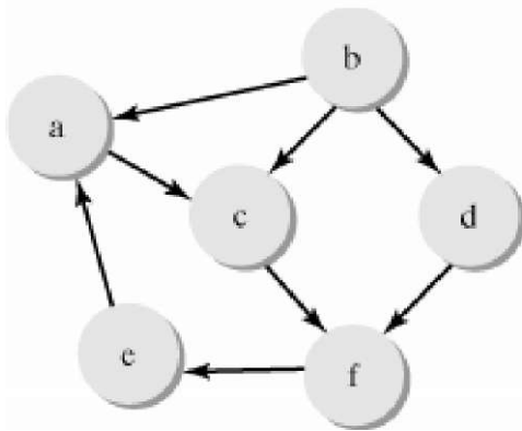
Рис. 3. Напрявлений граф.
