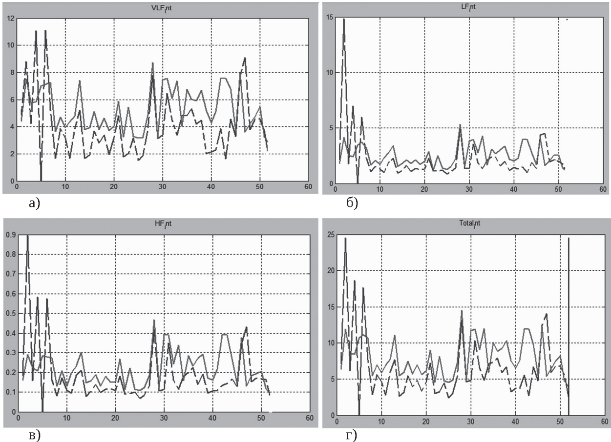
Рис. 2. Динаміка потужності спектру: а) VLFint, б) LFint, в) HFint, г) Totalint визначений у 55 обстежених до (переривчаста лінія) та під час (суцільна лінія) компресії плеча
