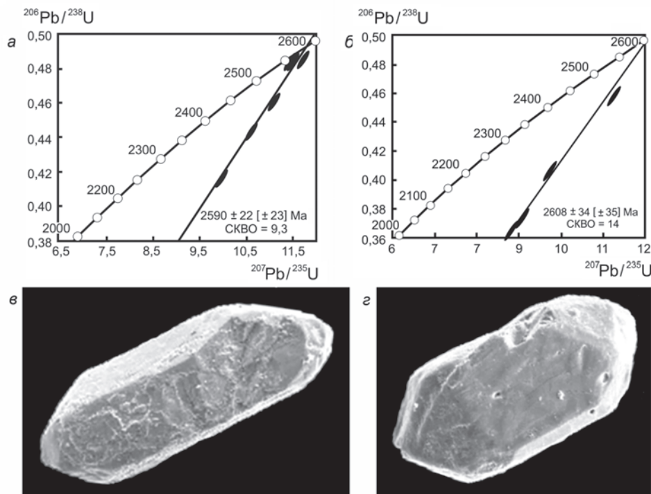
Рис. 6. Циркон із мігматиту порфірбластового тетівського комплексу: а, б — U-Pb ізохрони з конкордією (а — пр. ДЗ-5-1/84, б — пр. 0-1-84), в — пр. ДЗ-5-1/84, г — пр. 0-1-84
