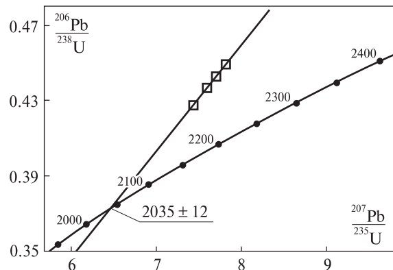
Рис. 6. U-Pb діаграма з конкордією для монацитів із мусковітізованого біотитового граніту, пр. К-1/3
