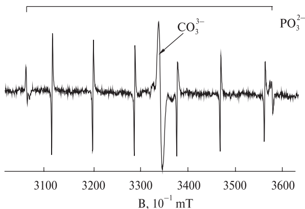
Рис. 4. Спектр ЭПР контрольного образца (с нулевым содержанием магния), обработанного при 900 °С. Запись проведена при СВЧ мощности 0,13 мВт. Шесть линий с обратной фазой в спектре принадлежат иону Mn^{2+} в эталонном образце MgO
