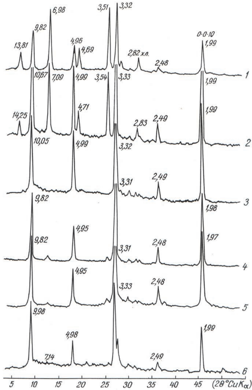
Рис. 8. Дифрактограми мусковіту і серициту з різних за складом порід: 1, 2 – серицит-хлоритові сланці; 3 – слюдяні пачки, що облямовують кварц-гранатове тіло; 4 – гранітогнейси; 5 – катаклазовані гранітогнейси.
