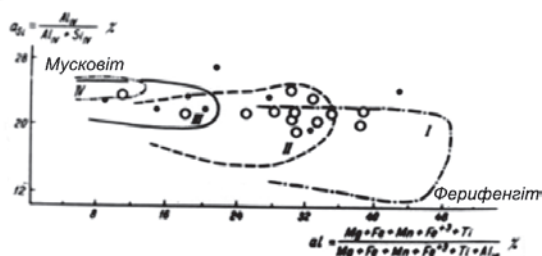
Рис. 4. Положення мусковітів білопотоцького (малі темні кружечки) і діловецького (великі порожні кружечки) на діаграмі a Si - a l , за [12]:
