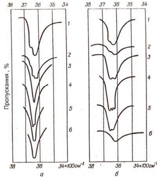
Рис. 10. ІЧ-спектри поглинання розтертих (а) і нерозтертих (б) мусковітів, за [9].
