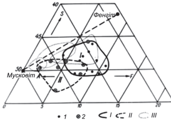
Рис. 5. Положення мусковітів з кристалічних порід на діаграмі ASF для серицит-мусковітів з метапелітів андалузит-силіманітового типу регіонального метаморфізму, за [3]:
