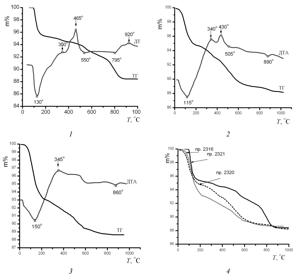
Рис. 2. Криві ДТА і ТГ водонерозчинного залишку гіпсів, фракція < 0,004 мм: 1 – пр. 2 321; 2 – пр. 2 320; 3 – пр. 2 316; 4 – криві втрати маси.
