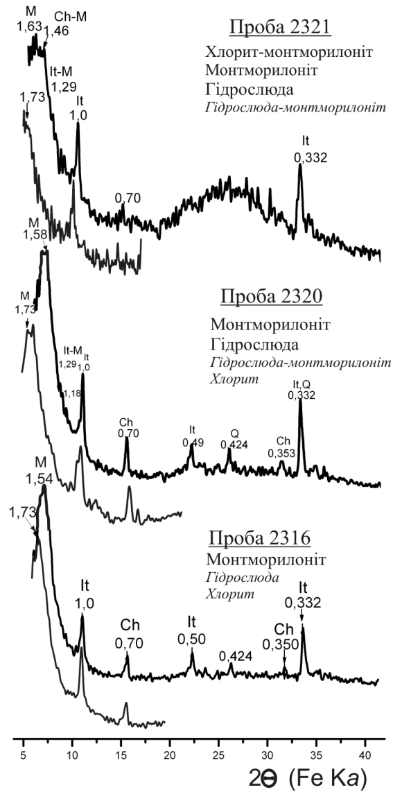
Рис. 1. Дифрактометричні криві та мінеральний склад водонерозчинного залишку гіпсів, фракція < 0,004 мм (орієнтований препарат).
