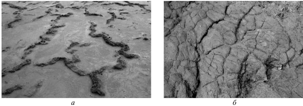
Рис. 4. Площинна ерозія поверхні хвостів флотажії, м. Стебник (а) та схилова ерозія поверхні солевідвалу № 2, м. Калуш (б).
