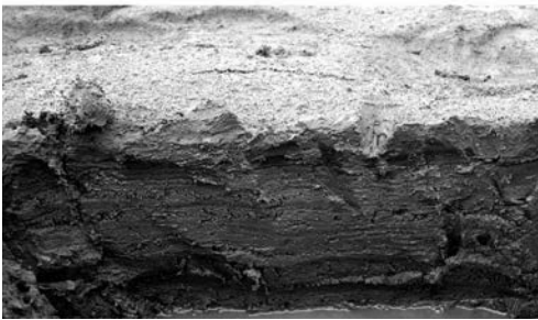
Рис. 13. Профіль гідроізоляційного глинистого прошарку в межах секції № 1 Стебницького хвостосховища.
