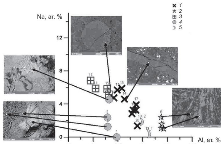
Рис. 7. Зміна співвідношення Al і Na як відображення перетворення смектит-хлорит.
