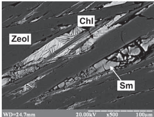
Рис. 8. Розвиток морденіту по смектиту в парагенезисі з хлоритом. Межа морденіт–хлорит індукційна. Св. 4 188, гл. 77 м. BSE-зображення.
