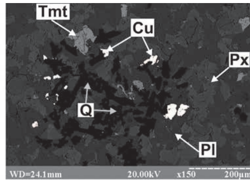
Рис. 12. Кварц-мідний дендрит, св. 4 188, гл. 77 м (а) та комп'ютерна обробка BSE-зображення (б).
