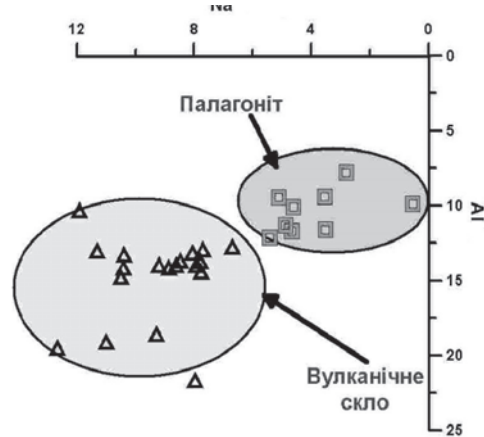
Рис. 3. Співвідношення Na і Al (ат. %) у вулканічному склі та палагоніті.
