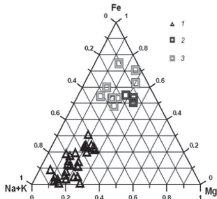
Рис. 2. Положення фігуративних точок складу вулканічного скла і палагоніту на трикутній діаграмі (Na+K)–Fe–Mg (AFM):
