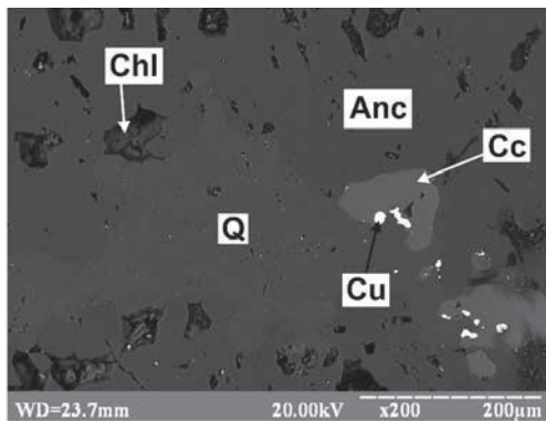
Рис. 15. Заміщення кальциту кварцом з самородною міддю. BSE-зображення.
