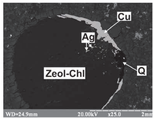
Рис. 14. Парагенезис самородної міді з кварцом і самородним сріблом у мигдалині, св. 4 188, гл. 77 м. Комп'ютерна обробка BSE-зображення.
