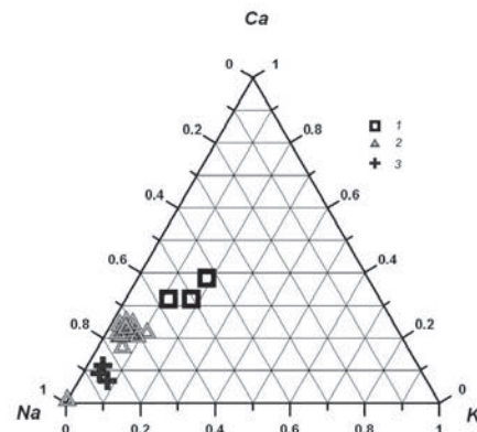
Рис. 9. Положення фігуративних точок складу морденіту на трикутній діаграмі Na–Ca–K. Взірці: 1 – св. 8 147, гл. 126,1 м; 2 – св. 8 262, гл. 289 м; 3 – св. 4 188, гл. 77 м.
