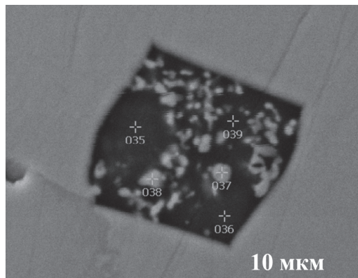
Рис. 6. Первинне включення у кристалі циркону з двома типами скла, що утворилися після нагрівання і загартування вмісту включення.
