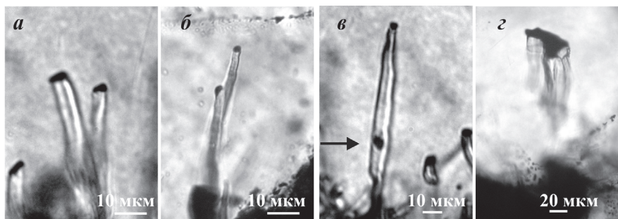
Рис. 4. Видовжені включення силікатного скла ( a–в ) та кальциту ( з ), вершини яких покриті пластинками самородного золота (чорні), у кварці Майського родовища золота (у прохідному світлі).
