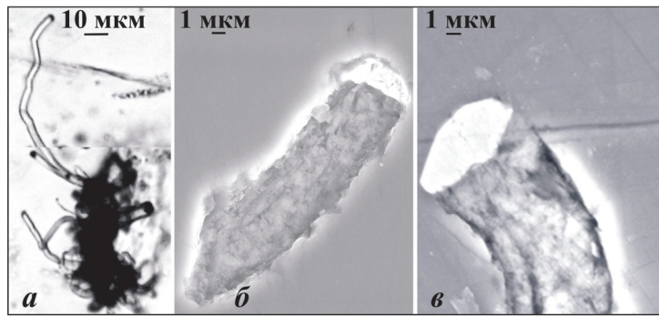
Рис. 3. Форма виділень силікатного скла у кварці апоскарнових кварцитів родовища Надія: a – загальний вигляд; б, в – деталі будови індивідів, вершини яких покриті пластинками, відповідно, самородного бісмуту й піротину; a – у прохідному світлі; б, в – РЕМ-зображення (сканувальний мікроскоп JSM-6700F).
