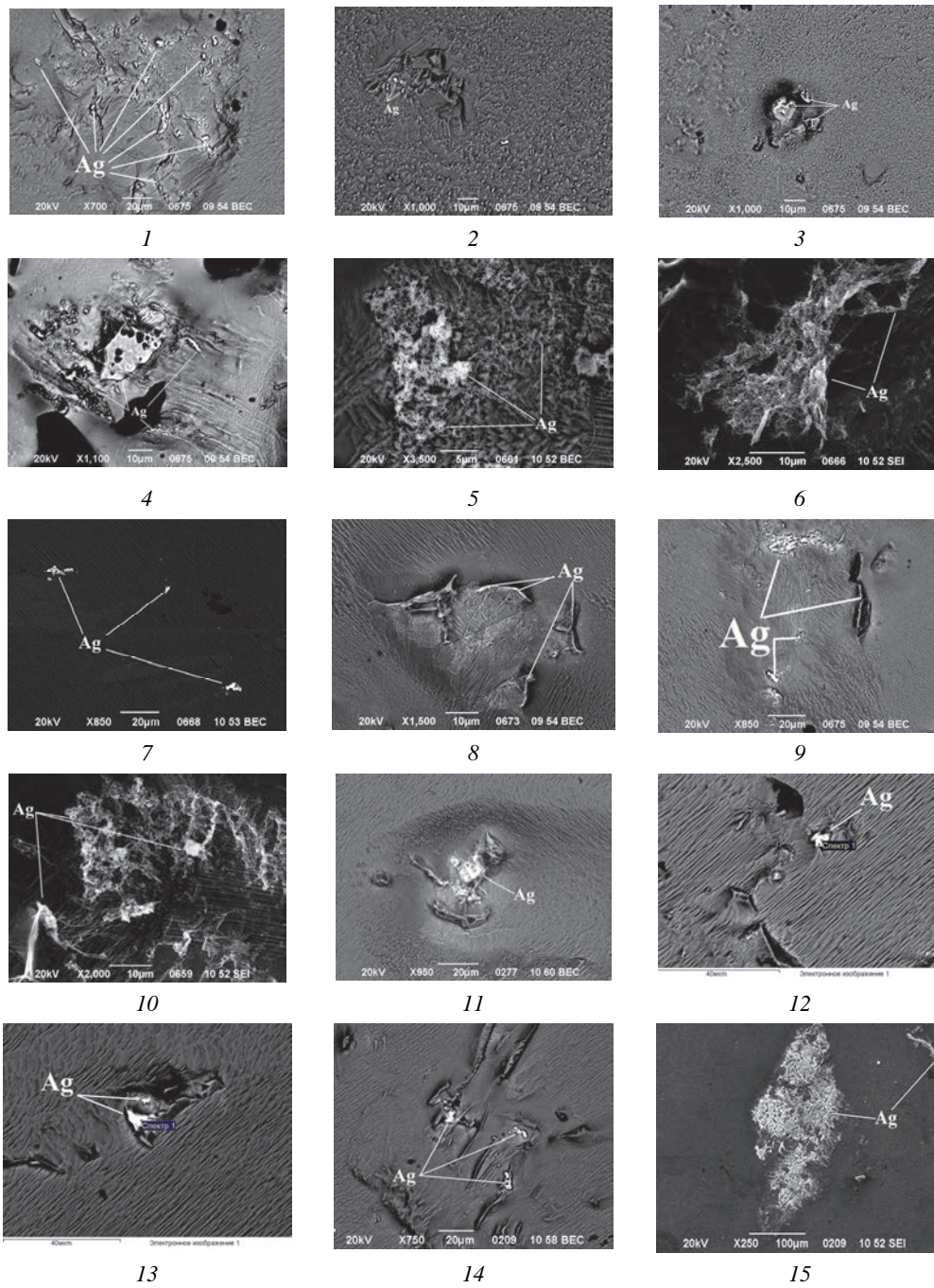
Рис. 3. Форми виділення самородного срібла (світле) на поверхні міді по зрізах:
