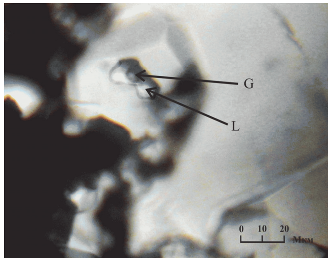
Рис. 2. Первинне газово-рідке включення у кристалику цеоліту (взірець 8273/17) з призальбандовій частині прожилка в базальті якушівської світи (зона зчленування Волинського палеозойського підняття і Волино-Подільської моноклінали): L – водний розчин, G – газова фаза; T_{\text{гом}} – 290 °С у рідку фазу.
