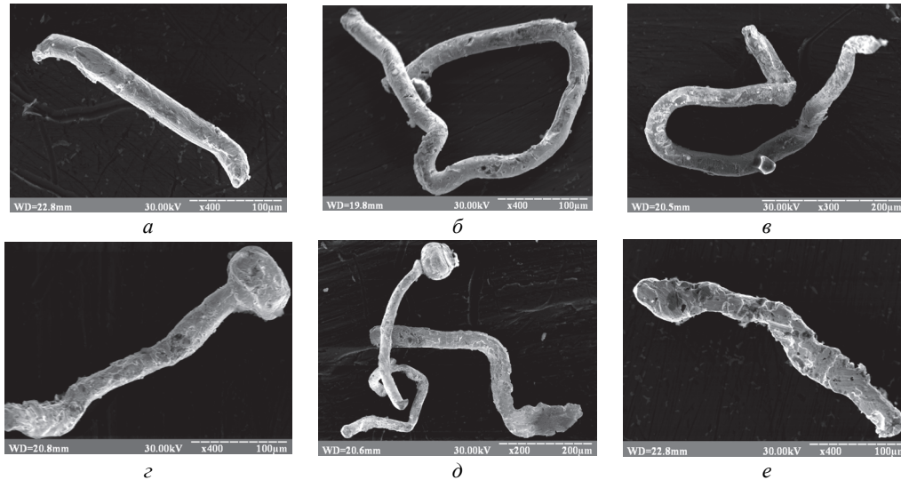
Рис. 2. Морфологія золота з крупнозернистих пісковиків:
