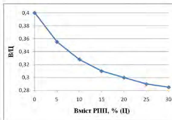
Рис.2. Вплив вмісту РПП на В/Ц рівнорухомої суміші (P=3,0 см)
