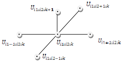
Рис 1. Явный шаблон конечно-разностной схемы для двухмерной задачи
