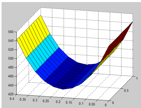
Рис. 2. Диаграмма распределения температуры по толщине слэба в момент времени равном 2400с
