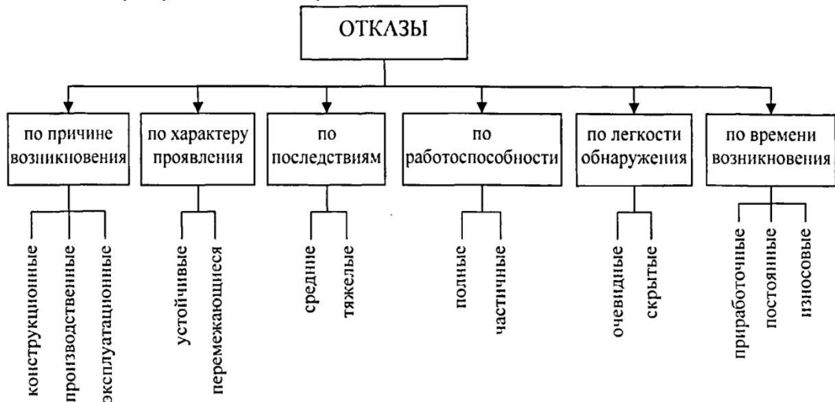
Рис. 1. Классификация отказов по признакам
