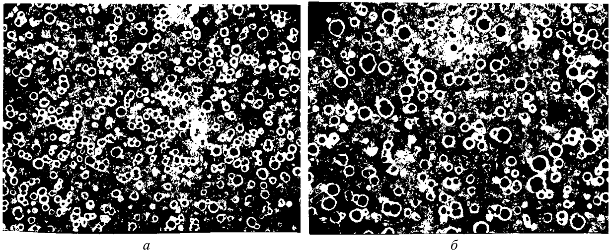
Рис. 2. Структура високоміцного чавуну, обробленого 0,4 % графітізуючого модифікатора оптимального складу у виливку з товщиною стінки: a — 6 мм, б — 16 мм × 200 мм
