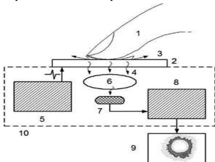
Рис. 2. Схематичне зображення ГРВ пристрою (1 – об'єкт дослідження; 2 - прозорий електрод; 3 - газовий розряд; 4 - оптичне випромінювання; 5 - генератор; 6 - оптична система; 7,8 – відеоперетворювач; 9 – комп'ютер; 10 – корпус)
