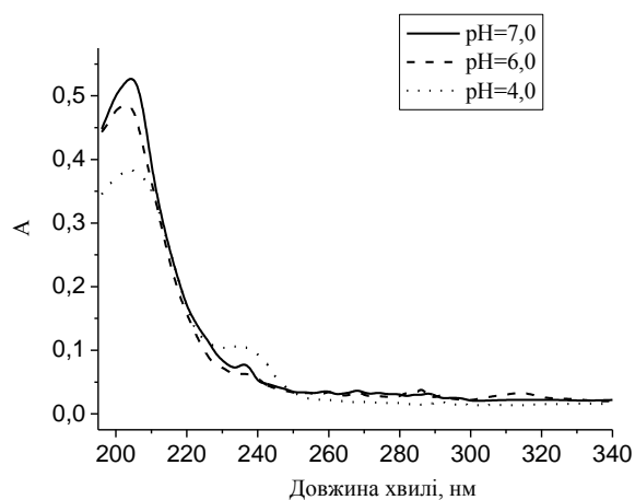
Рис. 2 Спектри поглинання розчинів меламіну при різних рН ( C_{\text{меламіну}}=1.0 \cdot 10^{-5} моль/л, l=1 см)
