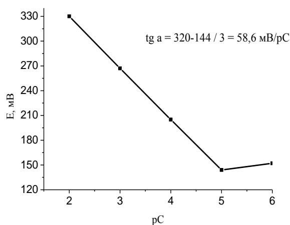
Рис. 9. Залежність потенціалу ICE від pC_{NH_4Cl}
