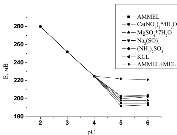
Рис. 8. Визначення потенціометричного коефіцієнту селективності K_{ij} ICE на амеліні методом змішаних розчинів у присутності заважаючих іонів.
