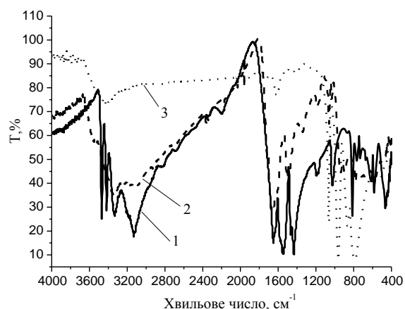
Рис. 5. ІЧ спектр поглинання: 1 – меламіну, 2 – МФК, 3 – сполуки MEL з PMo_{12}O_{40}^3 в таблетці KBr
