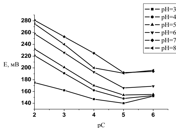
Рис. 7. Залежність потенціалу ICE від рС аммеліну при різних значеннях рН (мембрана з вмістом ЕАР 0.010 г; МР – ДБФ).
