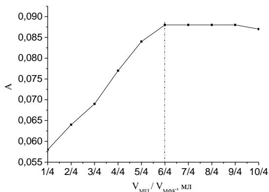
Рис. 4. Залежність поглинання системи MEL–МФК від концентрації меламіну ( V_{MFK}=4 мл; C_{MFK}=C_{меламіну}=10^{-5} моль/л, \lambda=236 нм; l=1 см)
