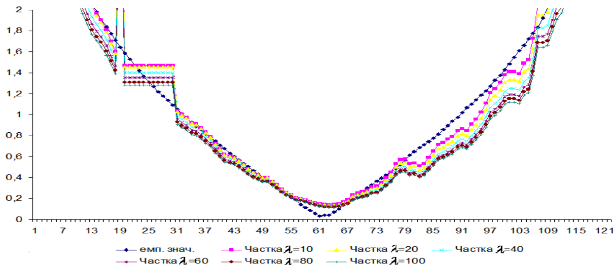
Рис.2. Тренд волатильності, як частки двох многочленів
