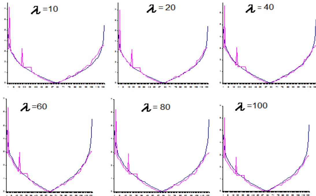
Рис.1. Квадратичний тренд при різних значеннях \lambda
