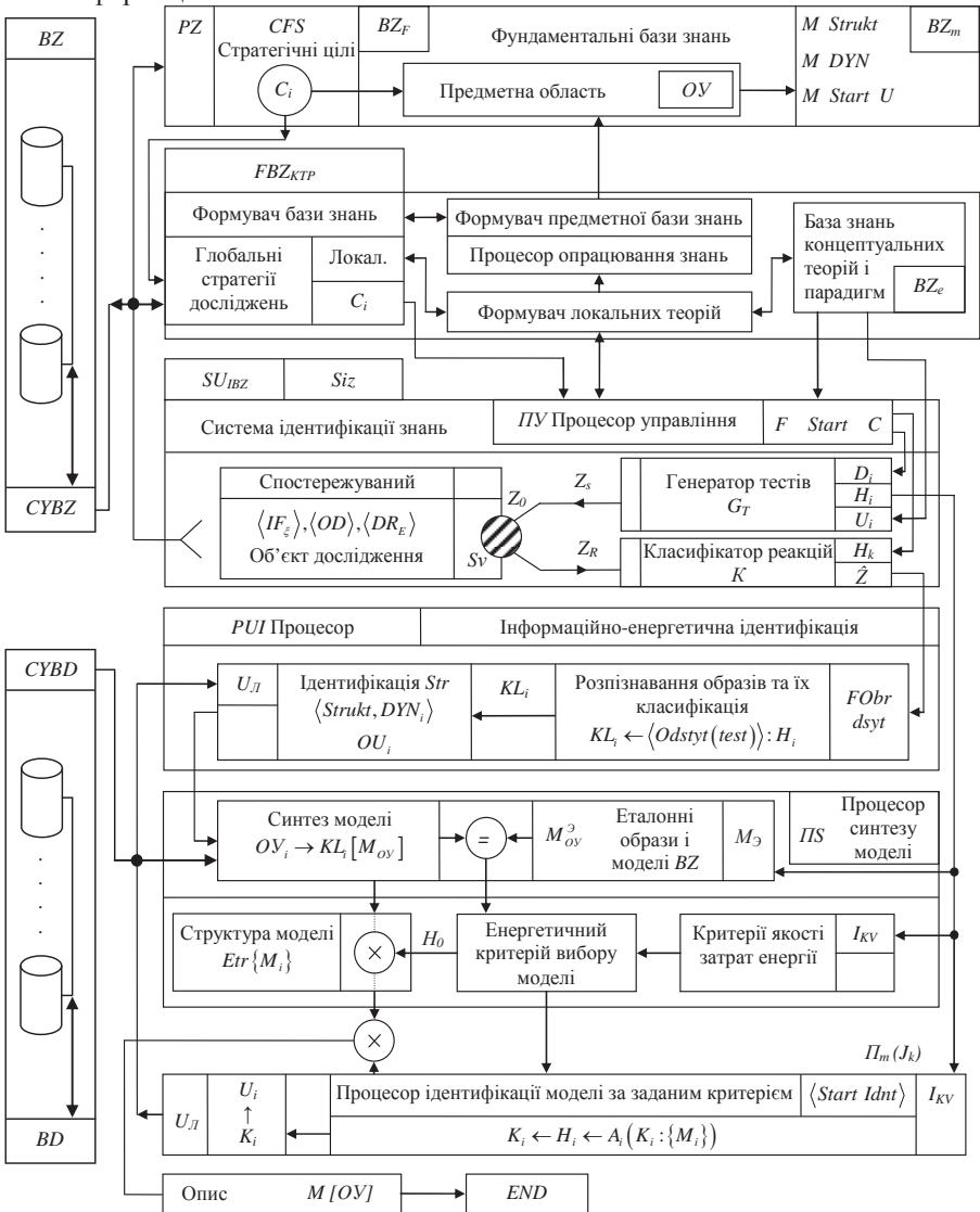
Рис. 2. Процедура вибору моделі структури системи гарантованого автоматичного управління (СГАУ) як основа для формування профорієнтованих базових тестів
