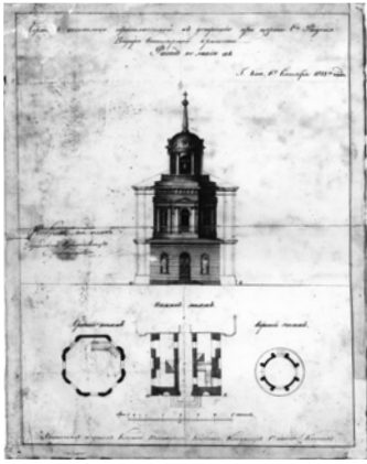
Станзані А. В. Проект дзвіниці церкви Феодосія Печерського, 1833 р. РДВІА, ф. 349, оп. 18,спр. 3109.
