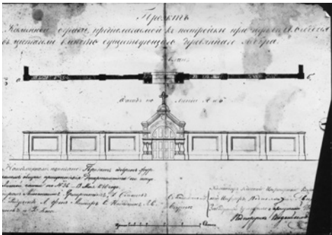
Проект кам'яної огорожі та воріт на подвір'ї церкви Феодосія Печерського, 1860 р.
