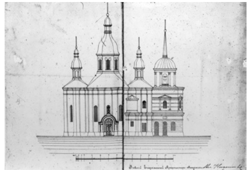
Архітектор Ніколаєв В. М. Проект пристосування холодної церкви в теплу та прибудова тамбура до церкви Феодосія Печерського, Фасад. 1896 р.
