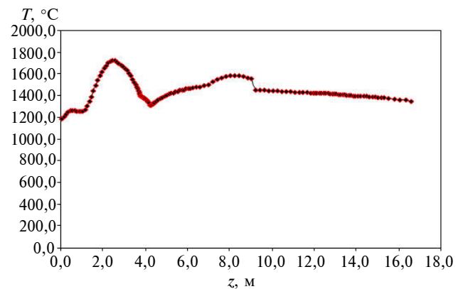
Рис. 9. Распределение температуры по высоте топочной камеры
