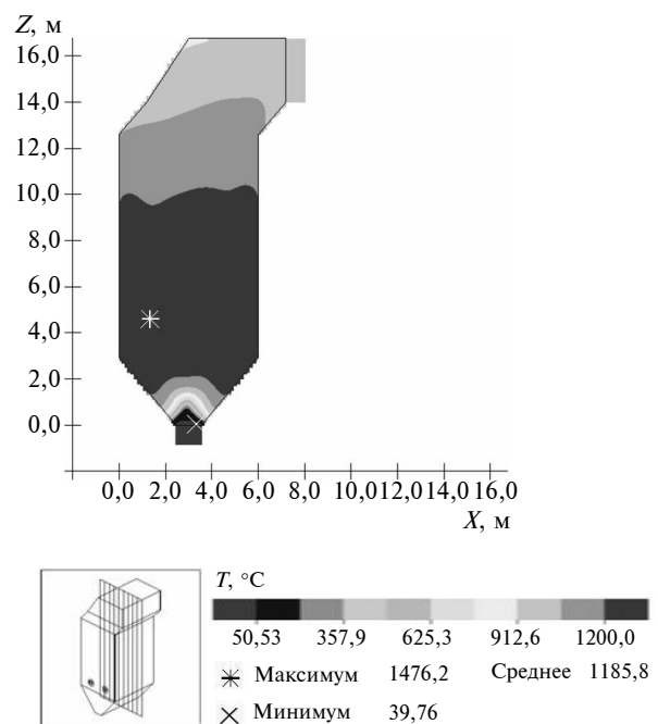
Рис. 8. Профиль температуры в области горелок и в продольном сечении камеры сгорания
