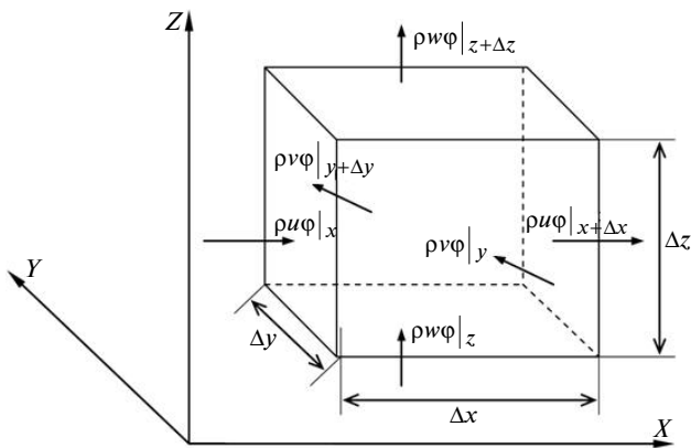
Рис. 1. Контрольный объем для обобщенного уравнения переноса [4], где \rho u \phi|_{i,i+\Delta i} описывает конвективный перенос транспортной переменной через границы контрольного объема в декартовой системе координат
