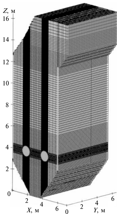
Рис. 3. Конечно-разностная сетка камеры сгорания БКЗ-75 Шахтинской ТЭЦ
