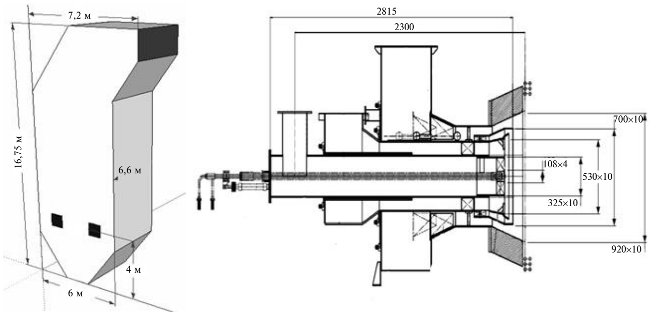
Рис. 2. Общий вид камеры сгорания и пылеугольной горелки
