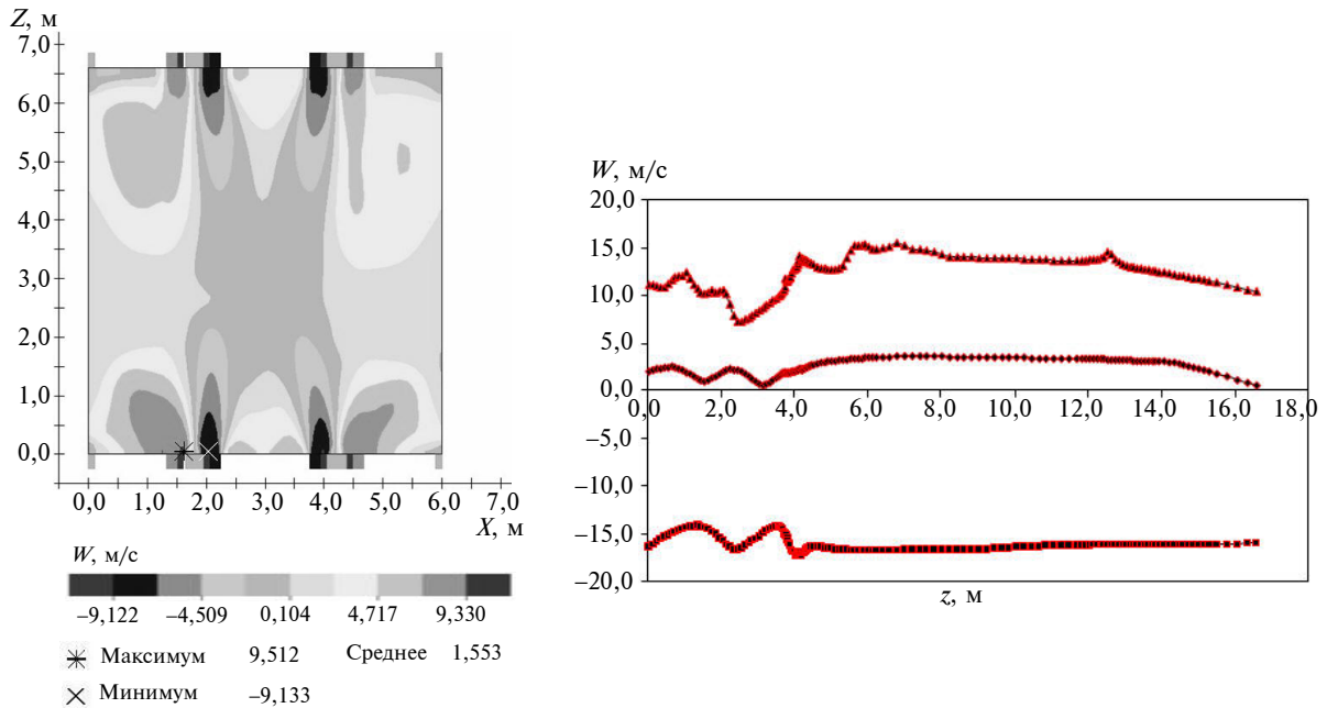
Рис. 6. Распределение составляющей скорости W в сечении горелок и по высоте камеры сгорания
