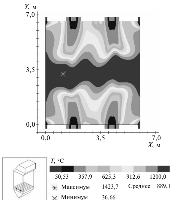
Рис. 8. Профиль температуры в области горелок и в продольном сечении камеры сгорания
