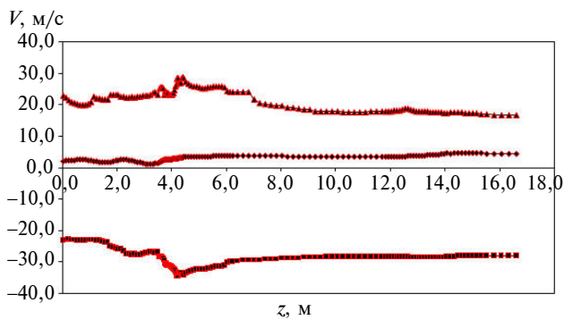
Рис. 7. Распределение вектора полной скорости по высоте камеры сгорания
