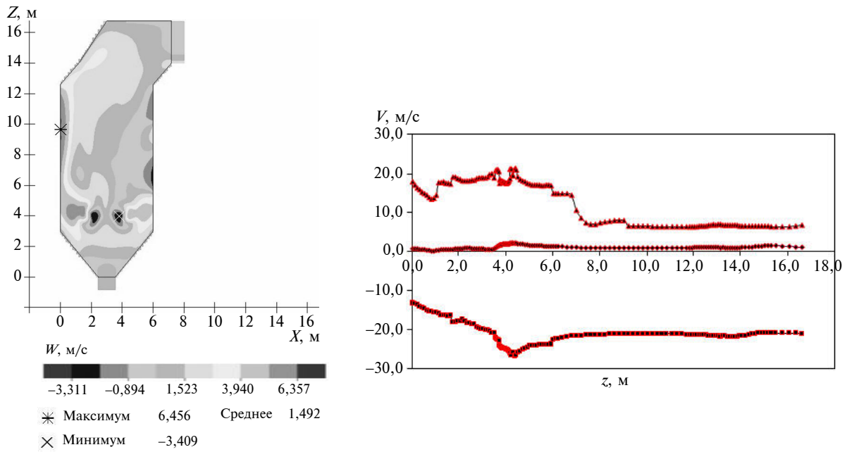
Рис. 5. Распределение составляющей скорости V в продольном сечении и по высоте камеры сгорания
