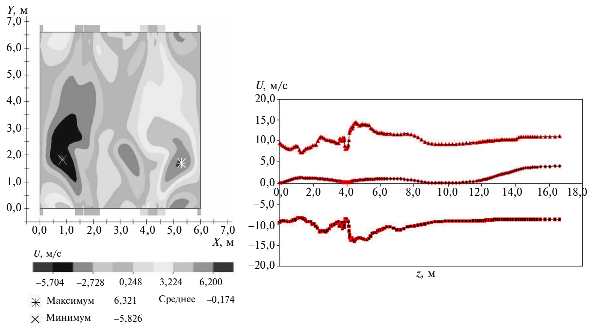
Рис. 4. Распределение составляющей скорости U в сечении горелки по высоте камеры сгорания; —●— среднее значение; —■— минимальное значение; —▲— максимальное значение
