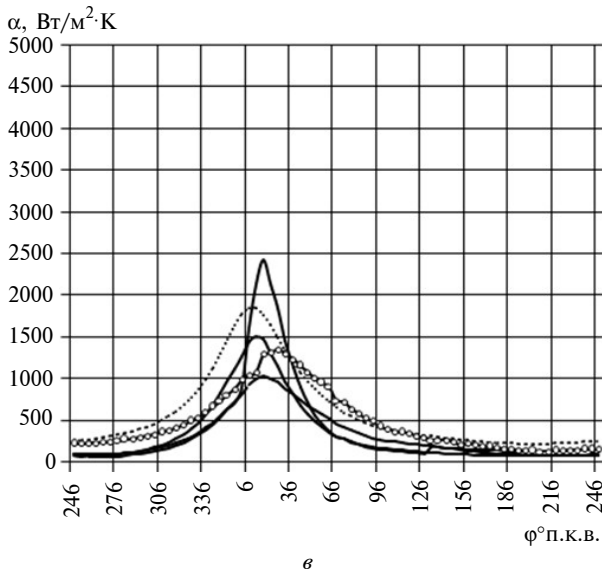
Рис. 4. Значення коефіцієнта тепловіддачі від газів до стінки надпоршневої поверхні циліндра, розраховані за різними формулами для визначення \alpha (% N_c ): а – 100; б – 75; в – 50; г – 25; — \alpha (Вошні); - - - \alpha (Ейхельберг); ..... \alpha (Аннанд); —○— \alpha (Розенбліт); - - - - \alpha (Хохенберг)
