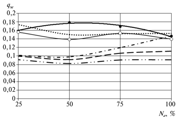
Рис. 5. Порівняння значень відносної втрати теплоти у стінки, розрахованої за різними формулами для визначення \alpha
