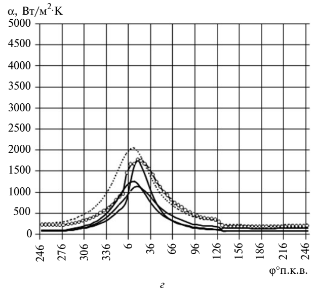
Рис. 4. Значення коефіцієнта тепловіддачі від газів до стінки надпоршневої поверхні циліндра, розраховані за різними формулами для визначення \alpha (% N_c ): а – 100; б – 75; в – 50; г – 25; — \alpha (Вошні); - - - \alpha (Ейхельберг); ..... \alpha (Аннанд); —○— \alpha (Розенбліт); - - - - \alpha (Хохенберг)
