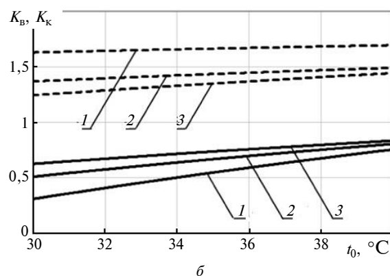
Рис. 3. Залежність частки повітря, що подається у конденсатор (----) та частки повітря, що подається у випарник (—) від температури навколишнього повітря при: а – \varphi = 60\% (1 – \Delta d_{2-1} = 1 \text{ г}_{\text{вл}} / \text{кг}_{\text{сп}} ; 2 – \Delta d_{2-1} = 2 \text{ г}_{\text{вл}} / \text{кг}_{\text{сп}} ; 3 – \Delta d_{2-1} = 3 \text{ г}_{\text{вл}} / \text{кг}_{\text{сп}} ); б – \Delta d_{2-1} = 2 \text{ г}_{\text{вл}} / \text{кг}_{\text{сп}} (1 – \varphi = 50\% ; 2 – \varphi = 60\% ; 3 – \varphi = 70\% )
