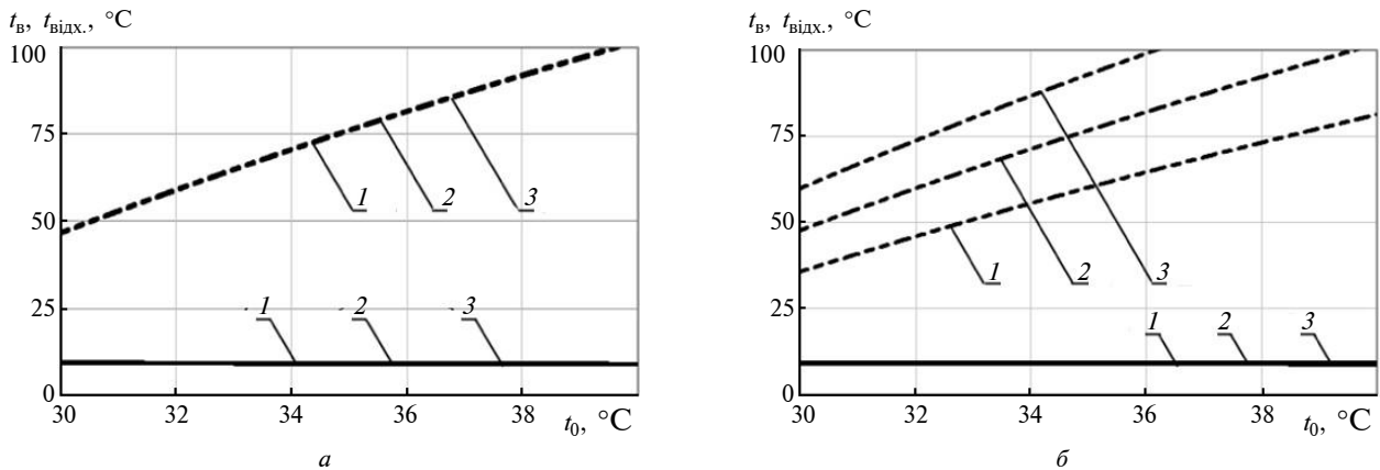
Рис. 4. Залежність температур повітря на виході із конденсатора ТН (----) та випарника ТН (—) від температури навколишнього повітря при: а – \phi = 60\% (1 – \Delta d_{2-1} = 1 \text{ г}_{\text{вл}} / \text{кг}_{\text{сп}} ; 2 – \Delta d_{2-1} = 2 \text{ г}_{\text{вл}} / \text{кг}_{\text{сп}} ; 3 – \Delta d_{2-1} = 3 \text{ г}_{\text{вл}} / \text{кг}_{\text{сп}} ); б – \Delta d_{2-1} = 2 \text{ г}_{\text{вл}} / \text{кг}_{\text{сп}} (1 – \phi = 50\% ; 2 – \phi = 60\% ; 3 – \phi = 70\% )
